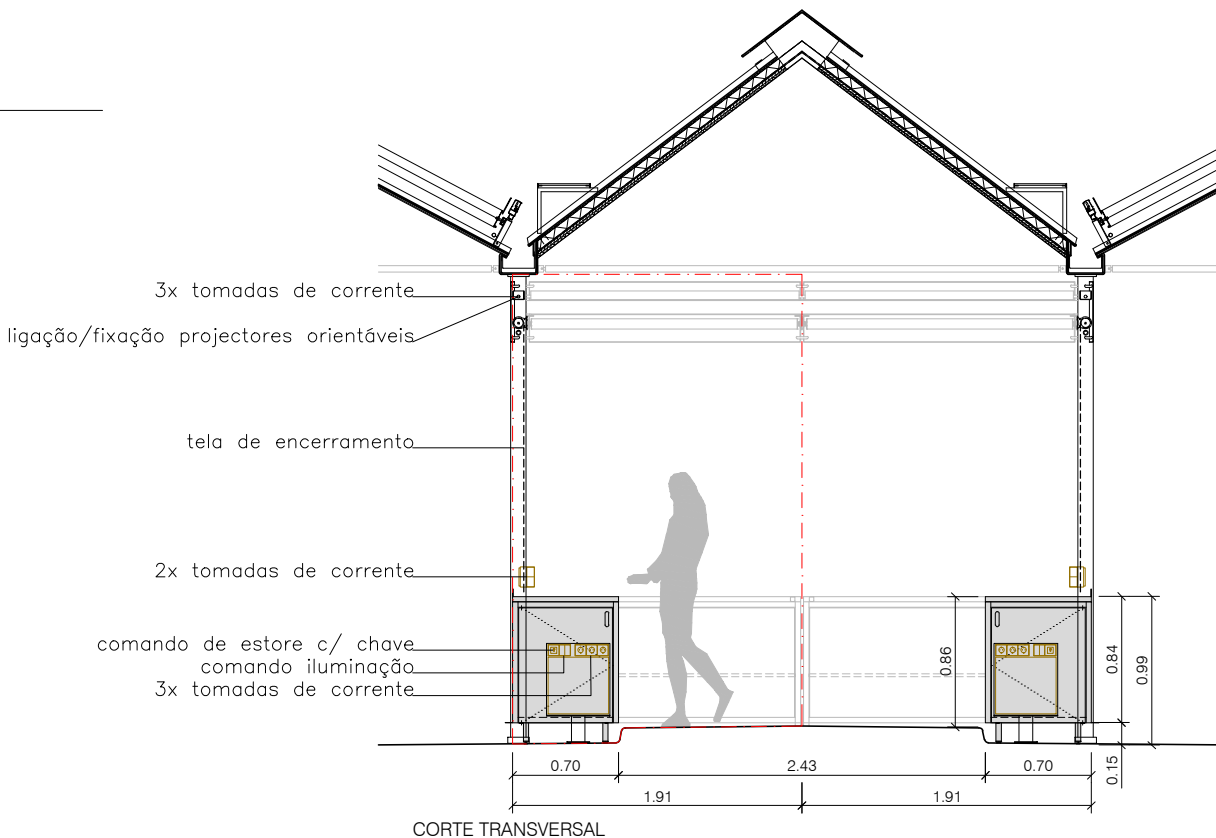
CORTE TRANSVERSAL
