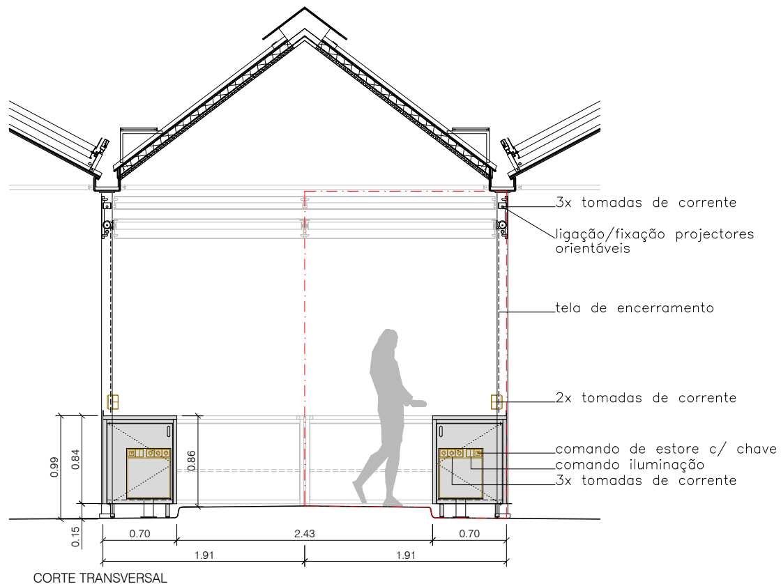
CORTE TRANSVERSAL
