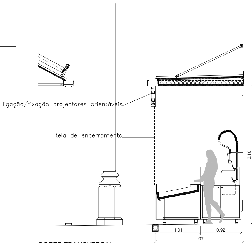
CORTE TRANSVERSAL
