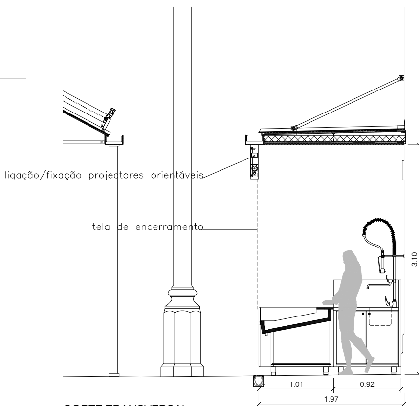
CORTE TRANSVERSAL
