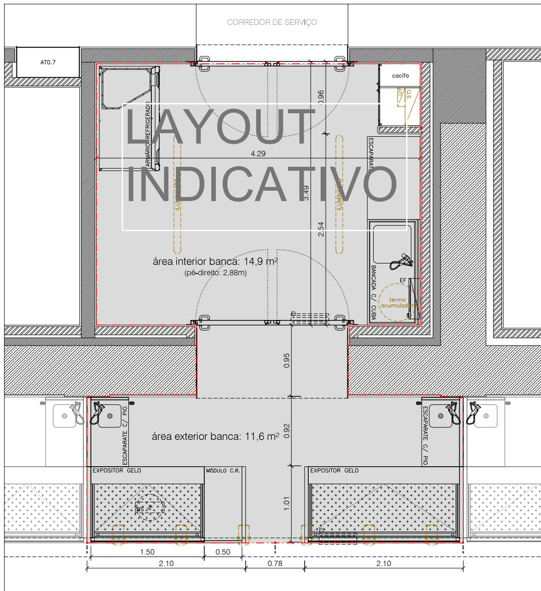
PLANTA
