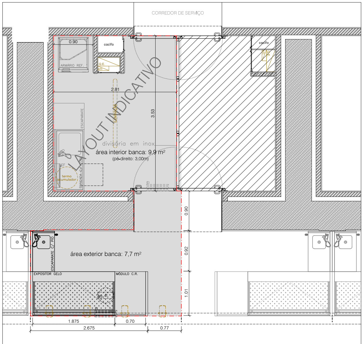
PLANTA
