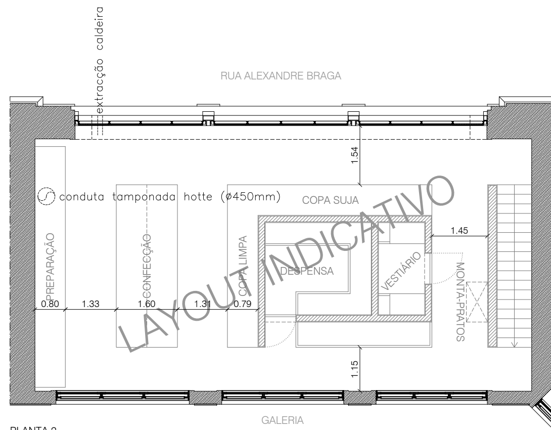
PLANTA 2 PISO SUPERIOR (a construir)
